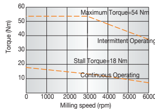
αiS 22/6000 (4.5 kW)
